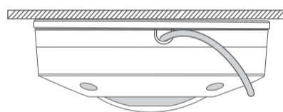
从侧面的走线孔走线
